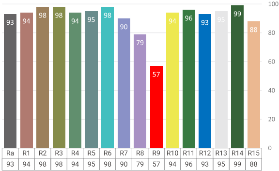
Min. Spot - 25°
