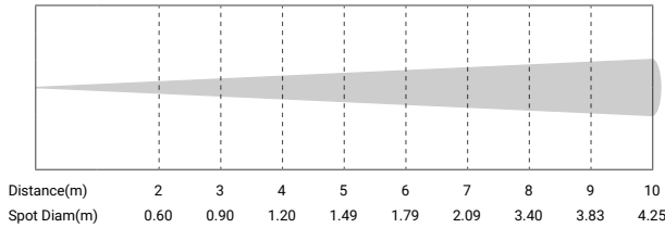
Min. Spot - 15°
