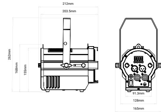
Min. Spot
